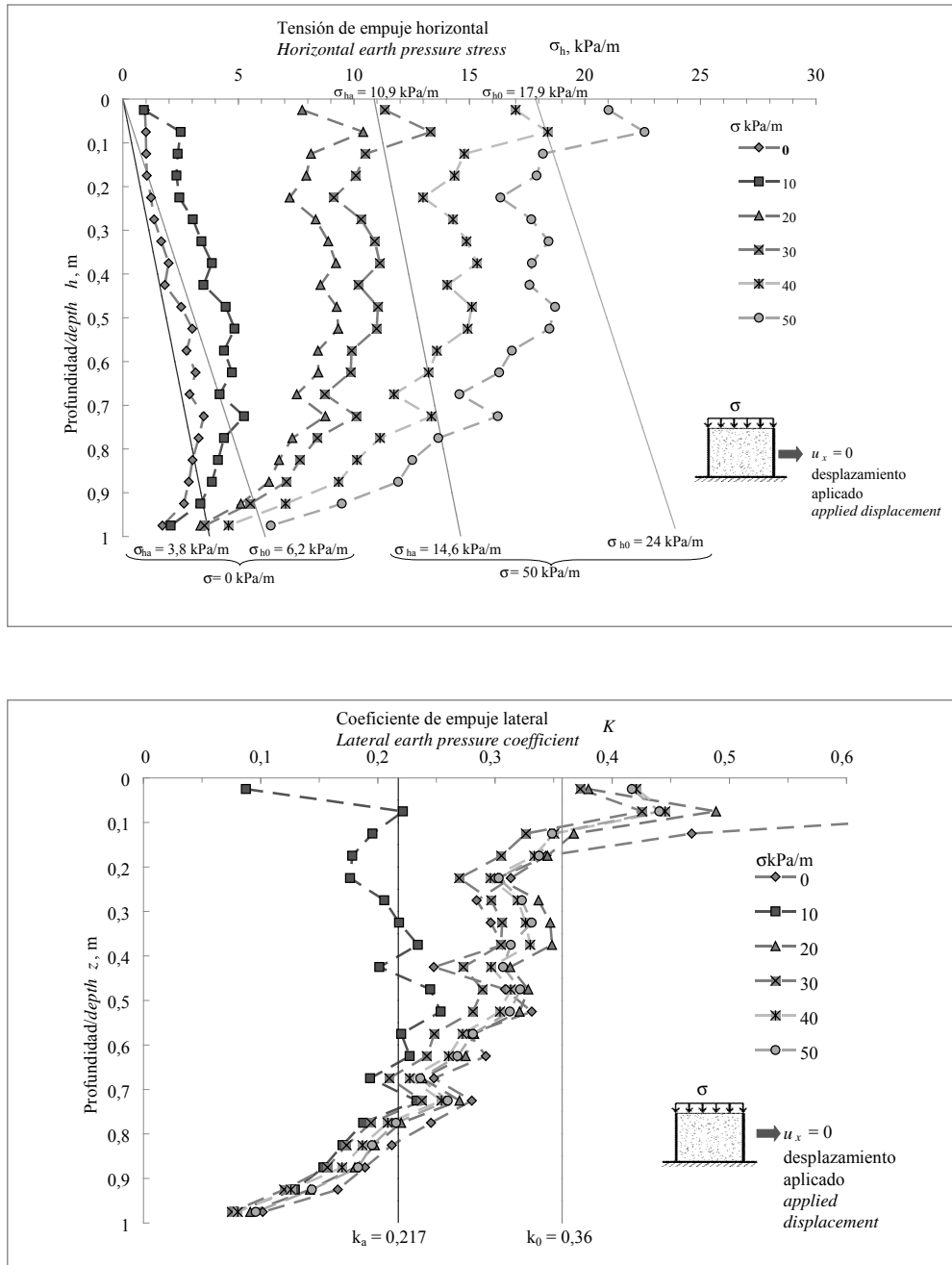
Figura 8. Suelo sin refuerzo; variación con la profundidad de a) la tensión de empuje horizontal y b) del coeficiente de empuje lateral, para el caso con u_x = 0 y \sigma variable
