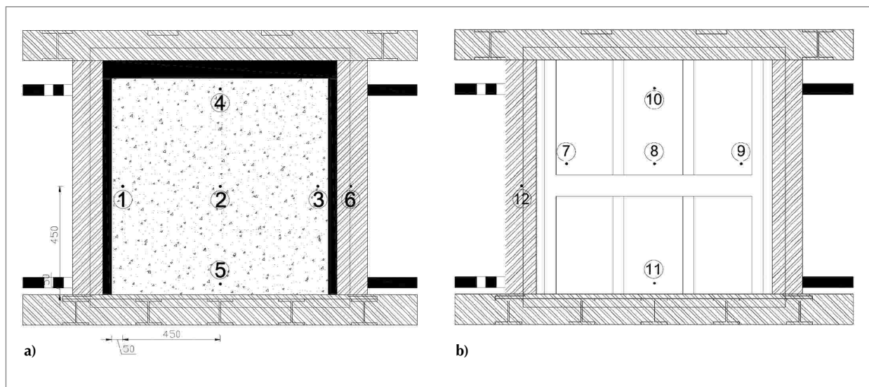
Figura 3. Disposición de los diales a) sobre la cara frontal de cristal y b) sobre la cara trasera de acero (dimensiones en mm) Figure 3. Dials arrangement a) over crystal front facing and b) over back steel facing (dimensions in mm)
