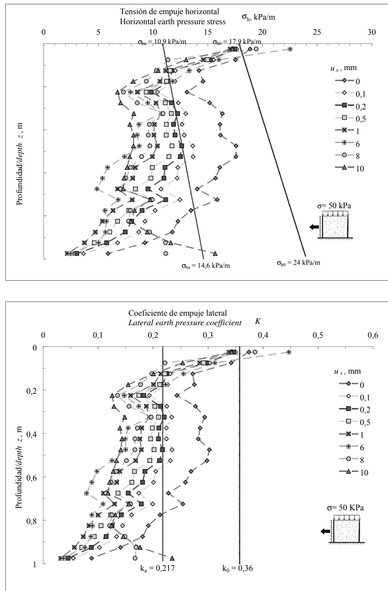
Figura 9. Suelo sin refuerzo; variación con la profundidad a) de la tensión de empuje horizontal y b) del coeficiente de empuje lateral, para el caso de \sigma = 50 kPa/m y u_x variable
