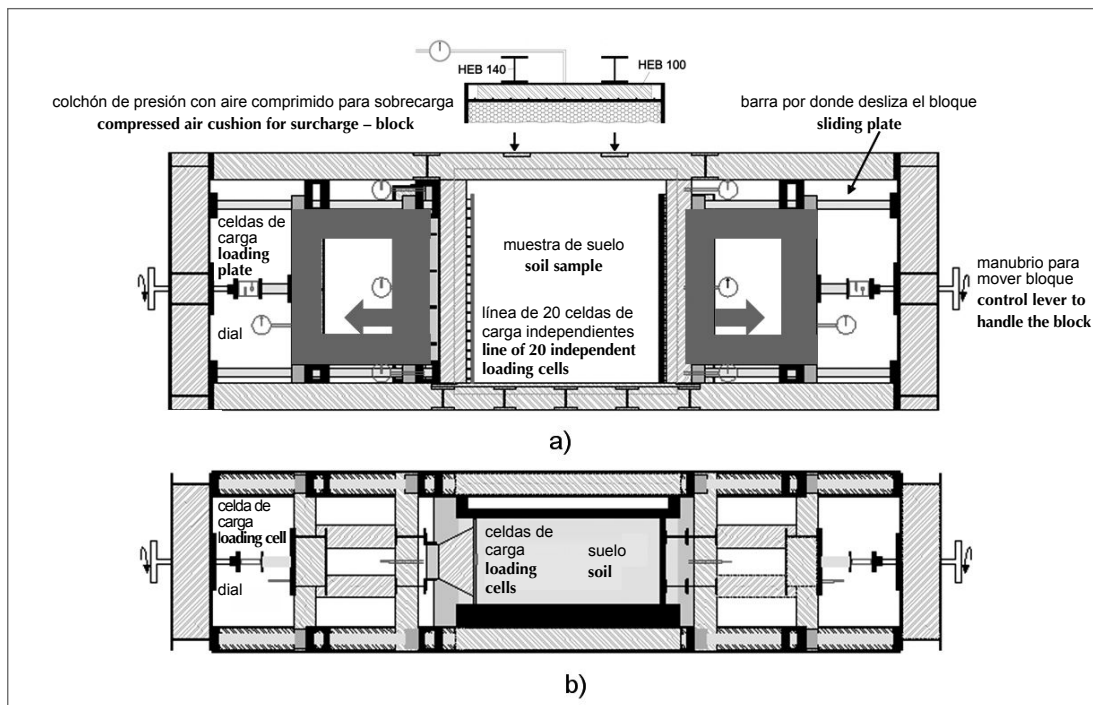
Figura 2. Esquema del equipo experimental: a) vista frontal y b) vista superior Figure 2. Experimental equipment sketch a) front view b) upper view
