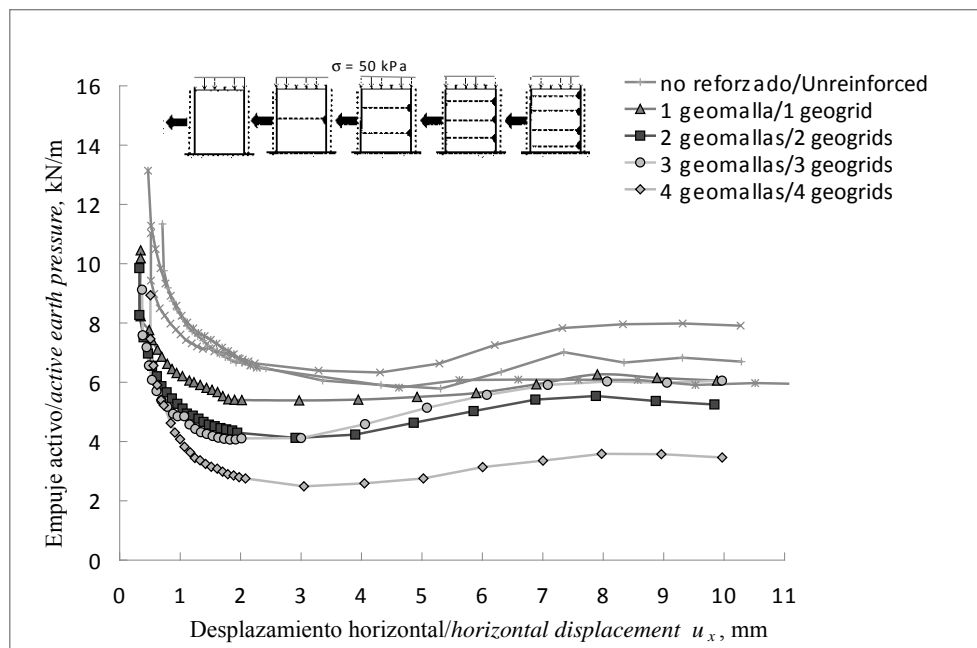
Figure 13. Variación de la fuerza de empuje versus el desplazamiento horizontal del muro para los casos sin y con varias geomallas de refuerzo
