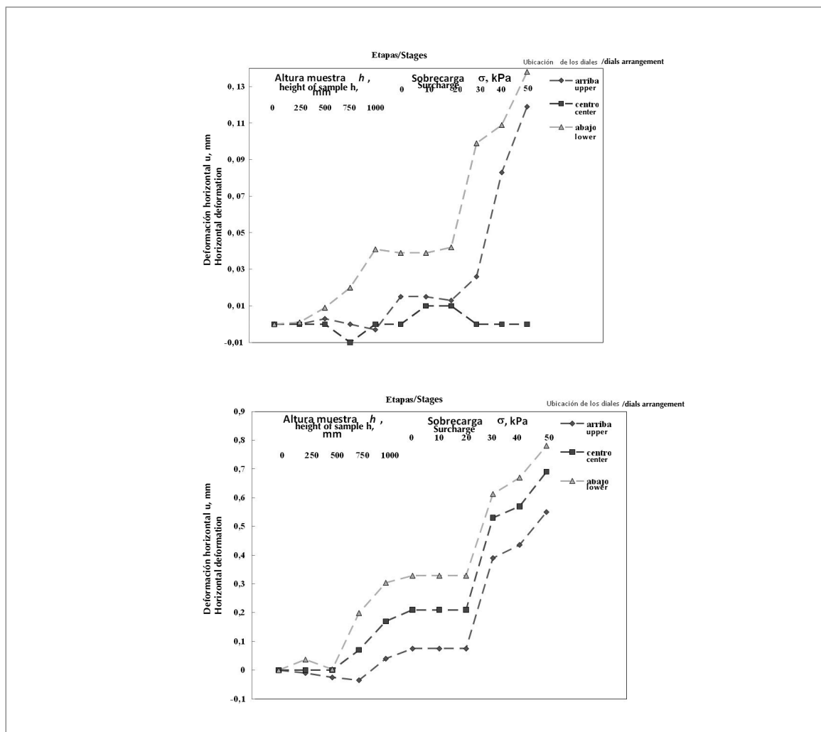
Figura 4. Deformación horizontal de las dos paredes móviles laterales durante el llenado y bajo sobrecarga Figure 4. Horizontal deformations on two mobile side walls during filling process and under surcharge condition
