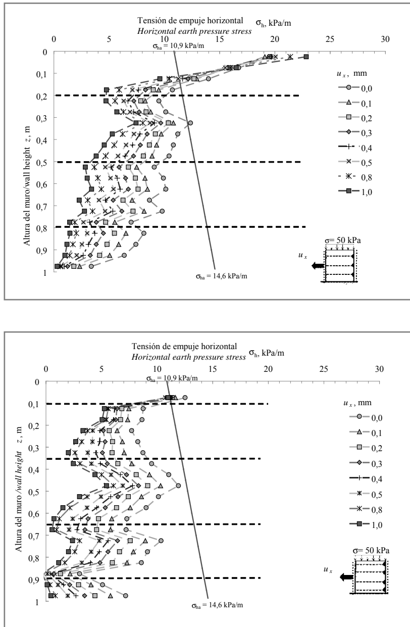
Figura 12. Variación de la tensión de empuje horizontal con la altura para suelo reforzado con a) tres y b) cuatro geomallas para el caso de \sigma = 50 kPa/m y u_x variable Figure 12. Variation of horizontal earth pressure stress versus height for a soil reinforced with a) three and b) four geogrids for the case of \sigma = 50 kPa/m and u_x variable
