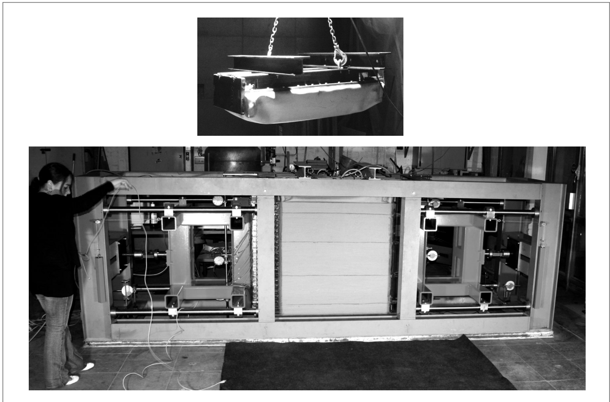
Figura 1. Vista frontal del equipo de ensayo con muestra preparada con 4 geomallas Figure 1. Front view of test apparatus including a sample prepared with 4 geogrids
