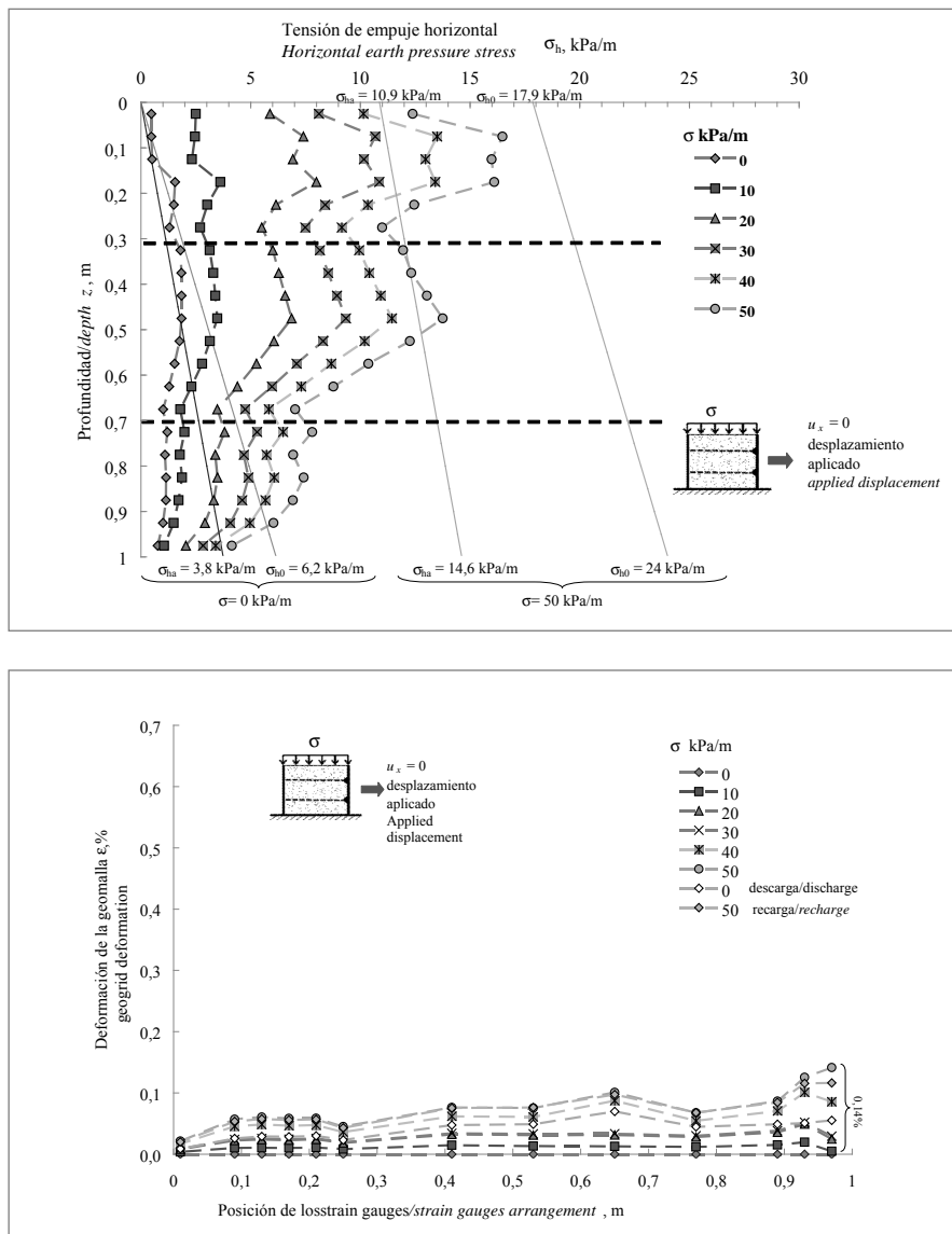
Figure 10. Suelo con dos geomallas de refuerzo; a) variación con la profundidad de la tensión de empuje horizontal y b) deformación de la geomalla superior en el plano horizontal para el caso de \sigma variable y u_x = 0 Figure 10. Soil reinforced with two geogrids a) variation with depth for horizontal earth pressure stress and b) upper geogrid deformation on a horizontal plane for the case \sigma variable and u_x = 0
