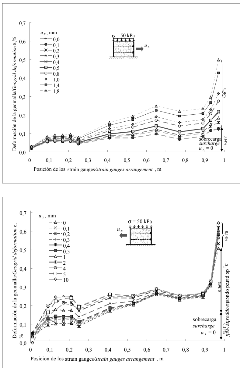
Figura 11. Suelo con dos geomallas de refuerzo; a) variación con la profundidad de la tensión de empuje horizontal, b) y c) deformación de la geomalla superior en el plano horizontal para el caso \sigma = 50 \text{ kPa/m} y u_x variable en ambas paredes Figure 11. Soil reinforced with two geogrids a) variation with depth for horizontal earth pressure stress b) and c) upper geogrid deformation on the horizontal plane for the case \sigma = 50 \text{ kPa/m} and u_x variable in both walls
