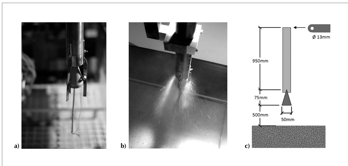
Figura 7. Dispositivo cónico móvil de control de riego de arena, esquema en c) no está a escala Figure 7. Mobile conic device to control sand pluviation; sketch on c) is not drawn to full scale
