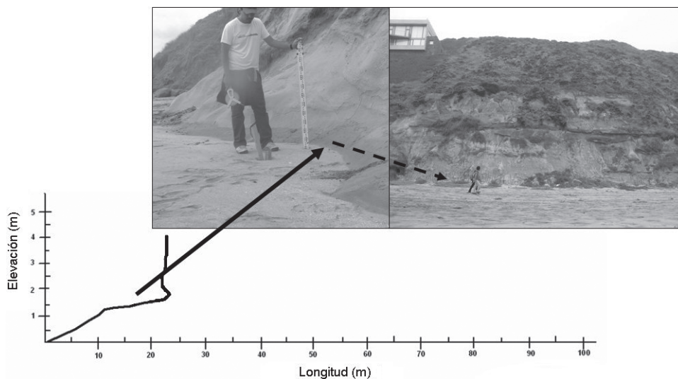
Figura N° 3 PLAYA DE CACHAGUA. PUNTO DE CONTROL CON MÁXIMA CONDICIÓN DE ATAQUE DEL OLAJE. LA MIRA TOPOGRÁFICA INDICA UNA ALTURA DE LA LÁMINA DE AGUA DE 23 CM COMO CONSECUENCIA DE LA EMBESTIDA DEL OLAJE, EN ENERO DE 2004. LA FOTO DE LA DERECHA CORRESPONDE A NOVIEMBRE DE 2006
