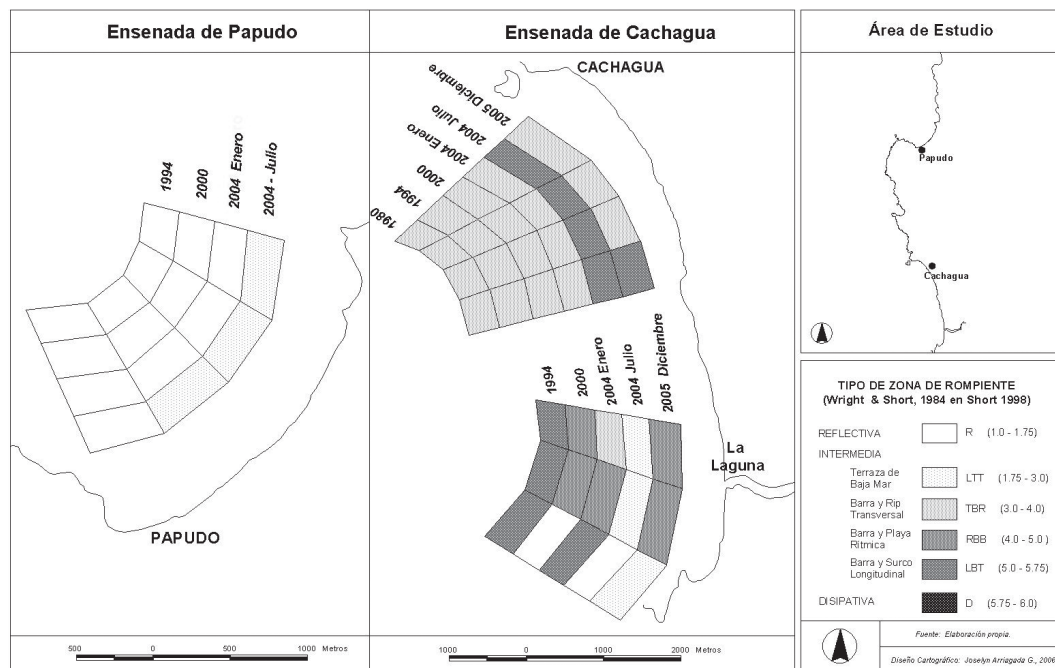
Figura N° 9 TIPOS DE ZONA DE ROMPIENTE, ENENADAS DE PAPUDO Y CACHAGUA
